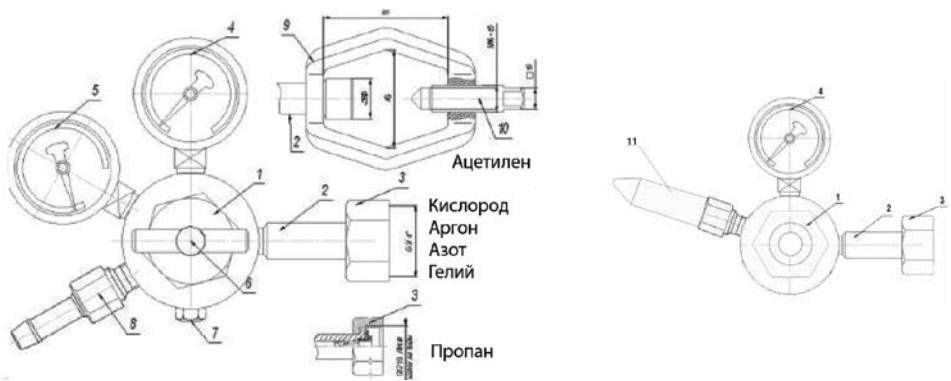
Рис. 1. Редуктор.
